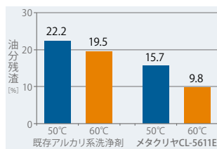
図2 洗浄試験
